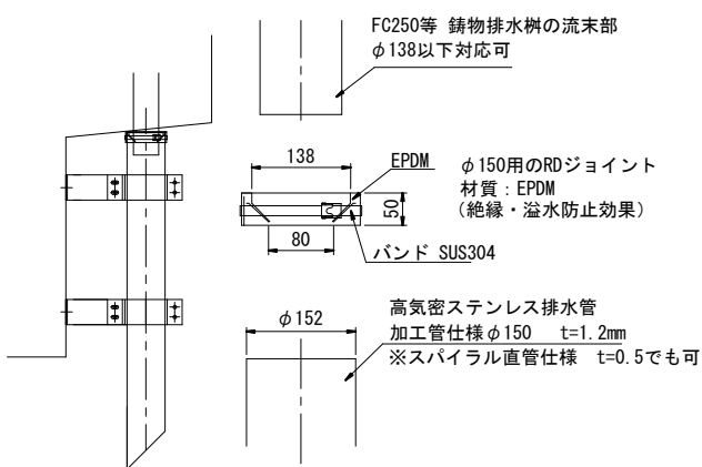
φ150用のRDジョイント使用例
