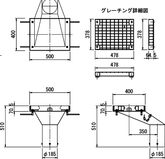
偏芯（中部地整）タイプ TSDR-GH
