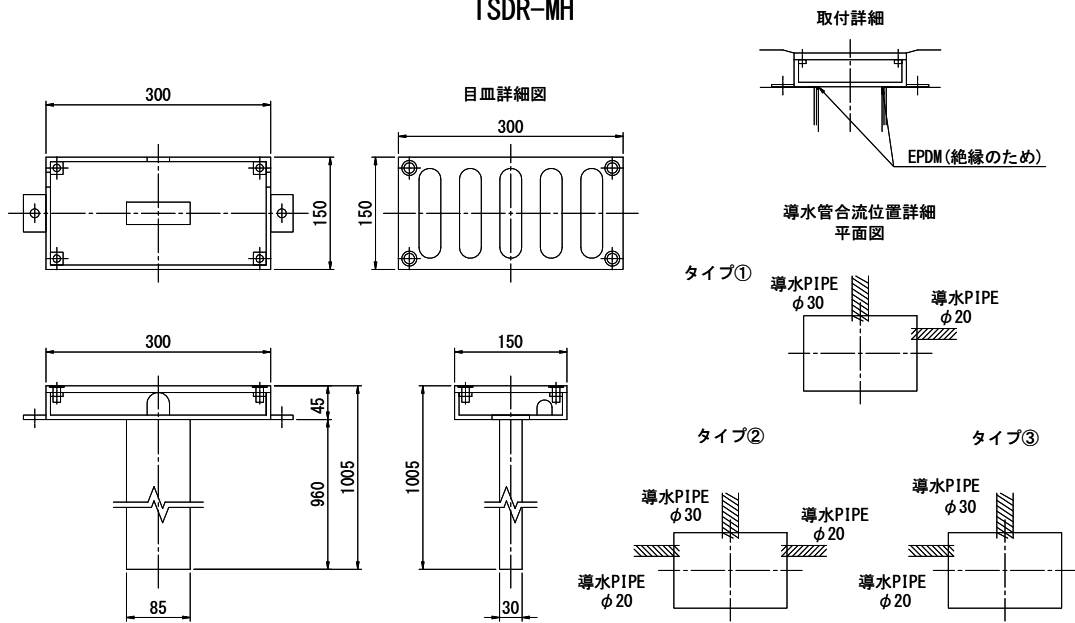
TSステンレス排水樹詳細図 TSDR-MH
