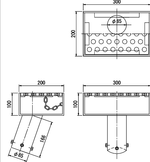
TSステンレス排水樹詳細図 TSDR-MH
