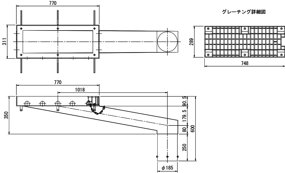
TSステンレス排水樹詳細図 TSDR-MH
