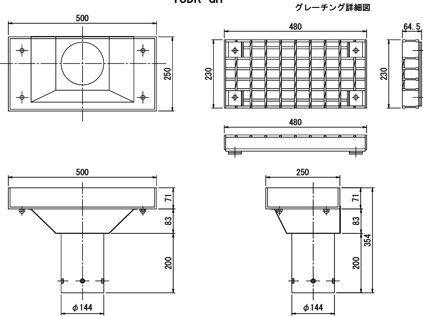
TSステンレス排水樹詳細図 TSDR-GH
