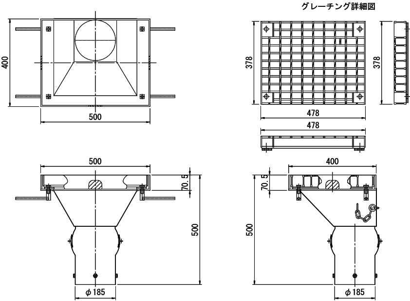
TSステンレス排水樹詳細図 TSDR-GH
