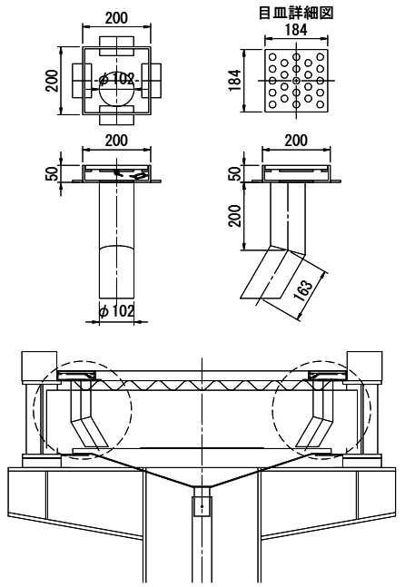
TSステンレス排水樹詳細図 TSDR-WH
