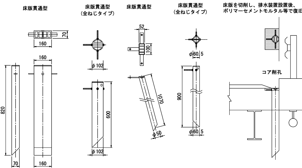
TSステンレス排水樹詳細図 TSDR-MH
