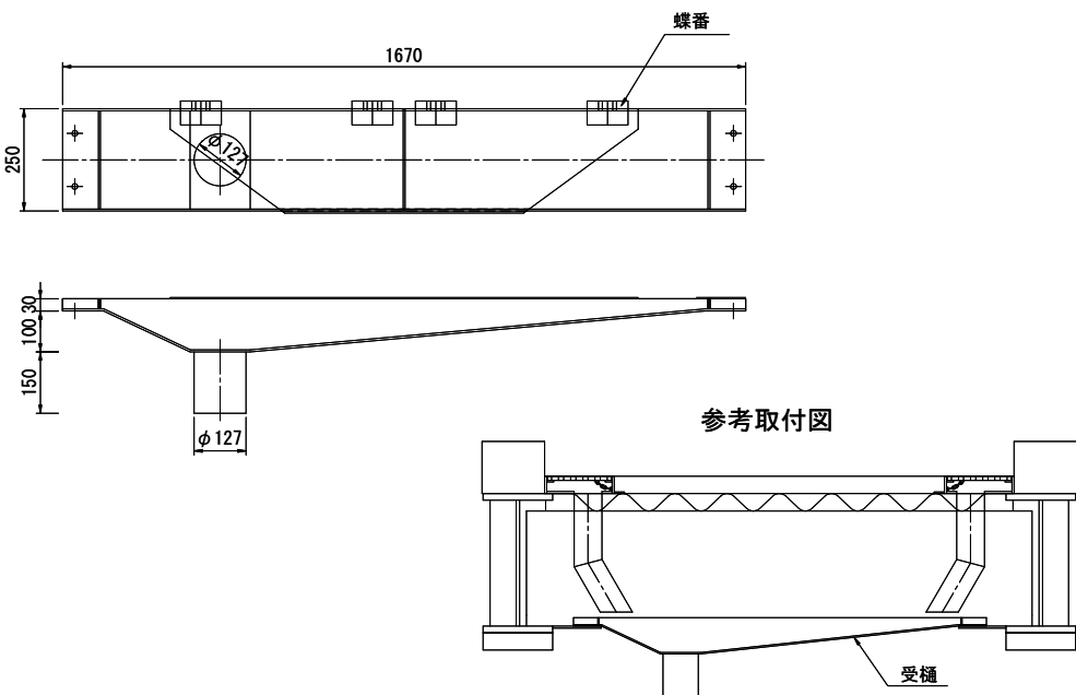
TSステンレス排水樹詳細図 TSDR-WU
