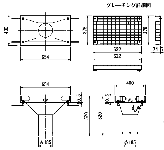
通常（近畿地整）タイプ TSDR-GH
