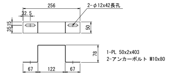
③取付金具詳細図 2組/セット
