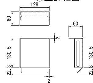
③取付金具詳細図 2組/セット
