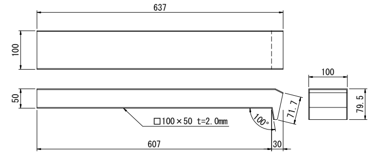
①横引詳細図
