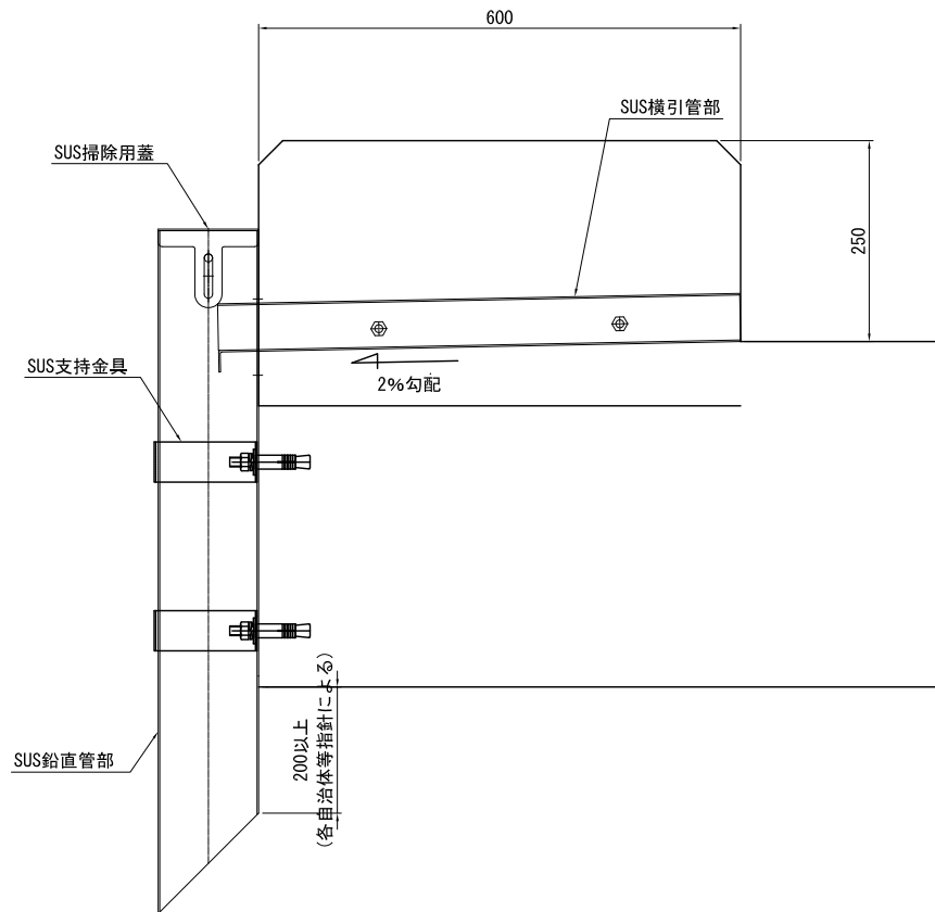
TSDR-SSD 設置例
