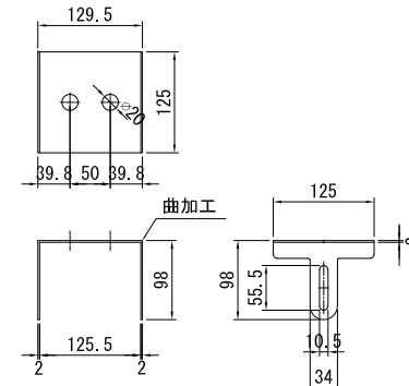
蓋詳細図
