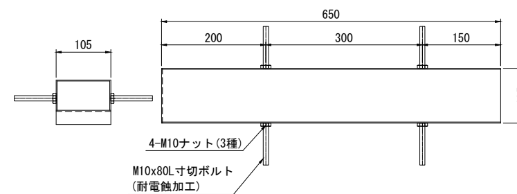
オプション2 寸切ボルト付
