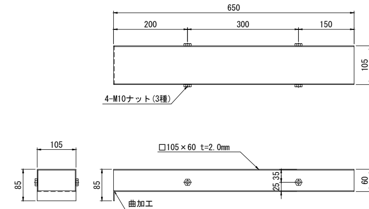
横引管部 詳細図
