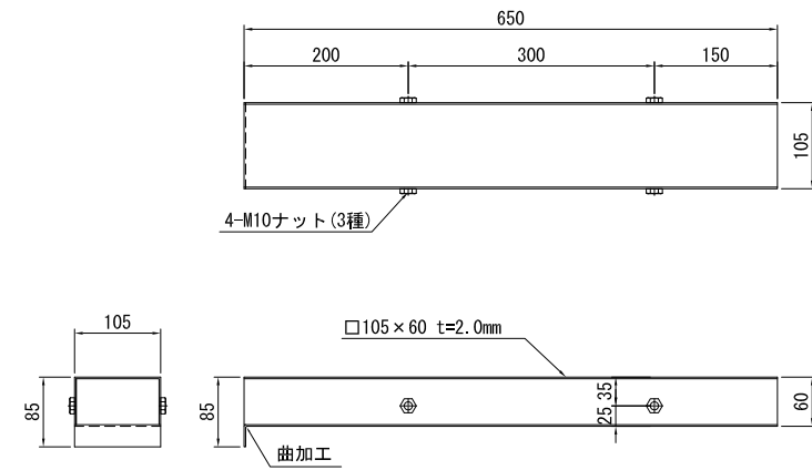
横引管部 詳細図
