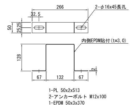
支持金具詳細図 2組/セット
