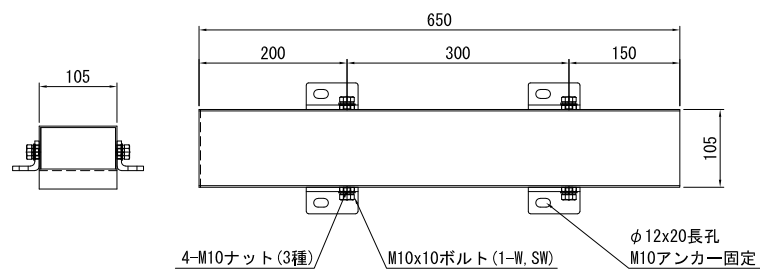
オプション1 アンカー固定用プレート付
