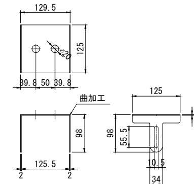
蓋詳細図
