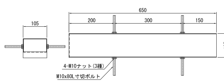
オプション2 寸切ボルト付
