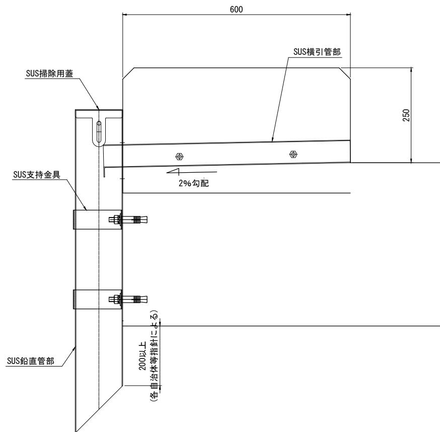
TSDR-SSD 設置例
