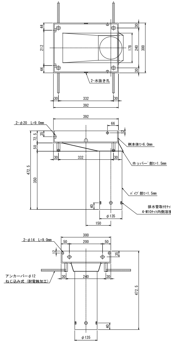
柵枠詳細図
