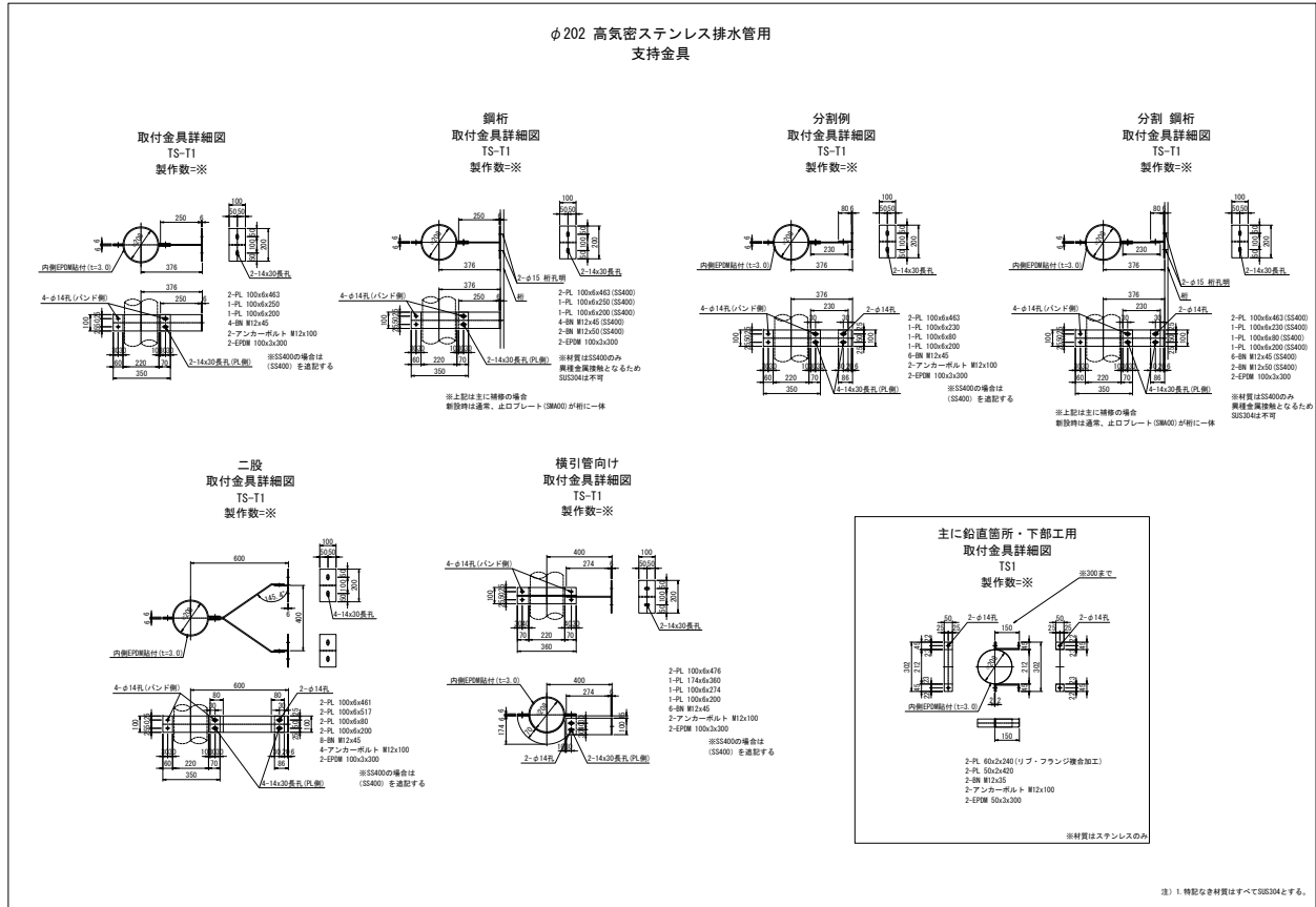
φ202 高気密ステンレス排水管用 支持金具 例
