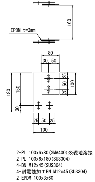
取付金具詳細図 TS-T1
