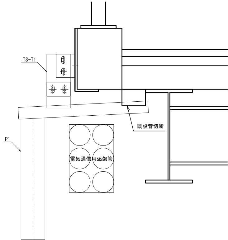
設置図
