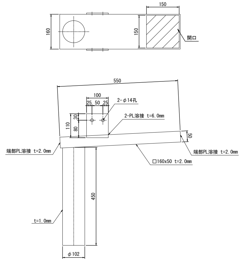
受け柵付排水管詳細図 P1
