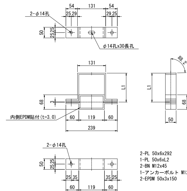
取付金具詳細図 B-1, 2, 3
