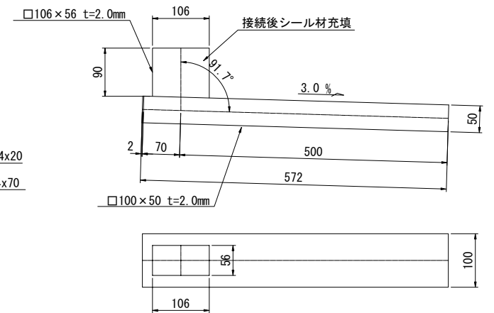
点検蓋詳細図
