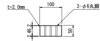
目皿詳細図
