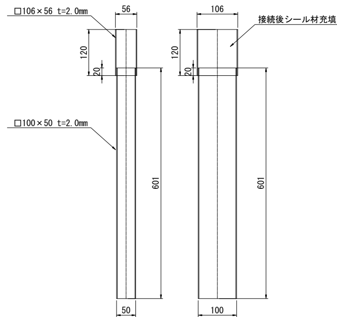
角管排水管 L2
