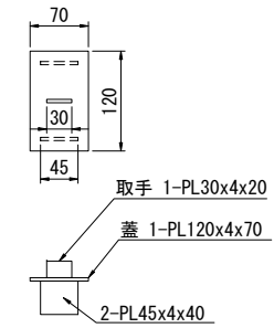
点検蓋詳細図
