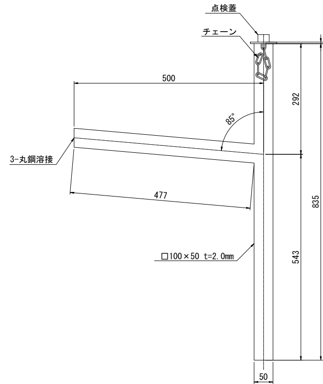
角管排水管 L3
