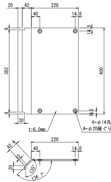
蓋詳細図 塗装色：日塗工 N-70 ライトグレー(蓋のみ)
